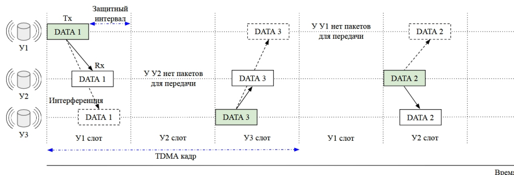
Рис. 2. Типовой пример мультиплексирования с временным разделением (TDMA), где каждому узлу назначается отдельный временной интервал для передач, при котором не происходит коллизий
